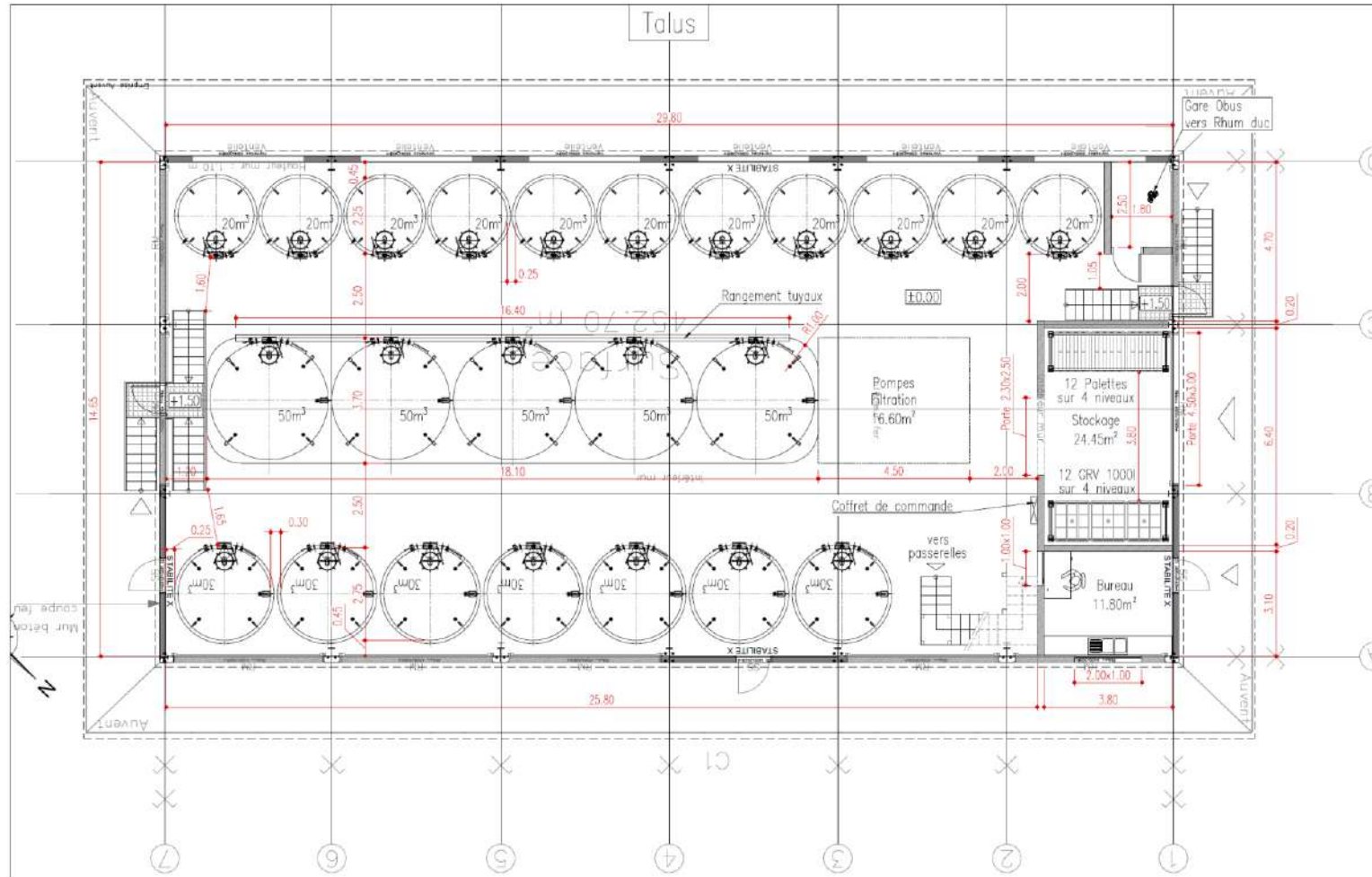
Plan de masse : Projet chai inox 2
