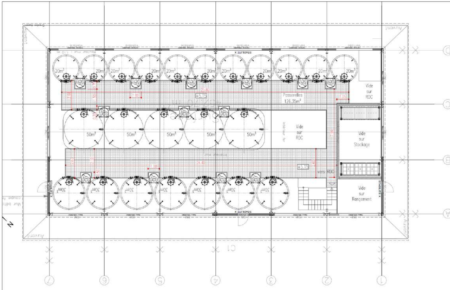
Plan de niveau : Projet chai inox 2
