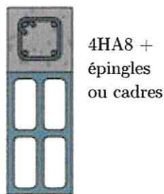
Exemple de coupe B-B
