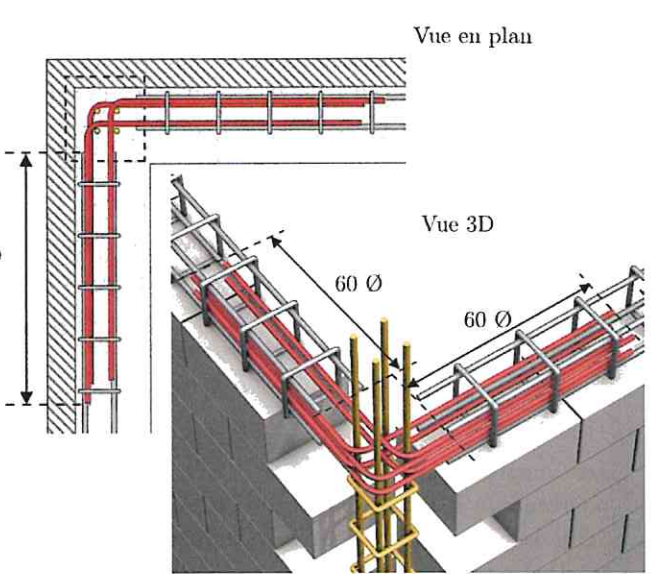
Liaison en angle avec équerres
