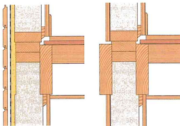
Détail 2-1
