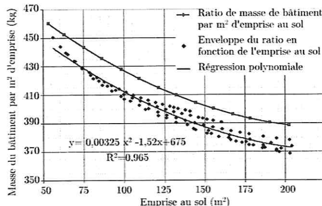
Figure D : évaluation de la masse par m² d'emprise au sol pour une construction en R+1 avec une toiture lourde
