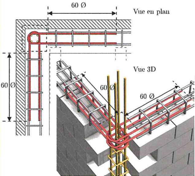
Liaison en angle avec boucles
