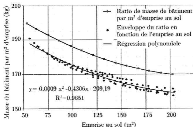
Figure C : évaluation de la masse par m² d'emprise au sol pour une construction en simple rez-de-chaussée avec une toiture lourde
