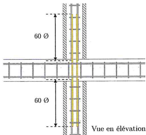
Chaînage au niveau d'un plancher
