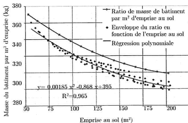
Figure B : évaluation de la masse par m² d'emprise au sol pour une construction en R+1 avec une toiture légère
