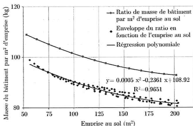
Figure A : évaluation de la masse par m² d'emprise au sol pour une construction en simple rez-de-chaussée avec une toiture légère
