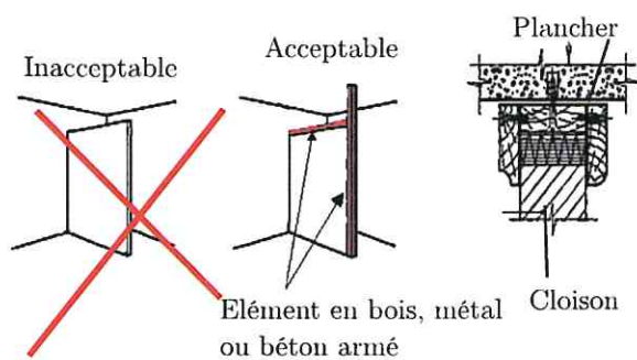
NOTE 115 - disposition des cloisons
