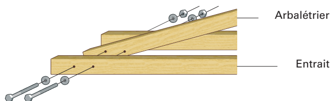
Figure 27 : Fiabilisation d'assemblage entrain moisé - arbalétrier par 2 boulons
