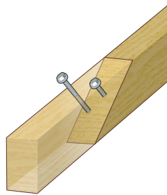
Figure 9 : Jonction vissée
