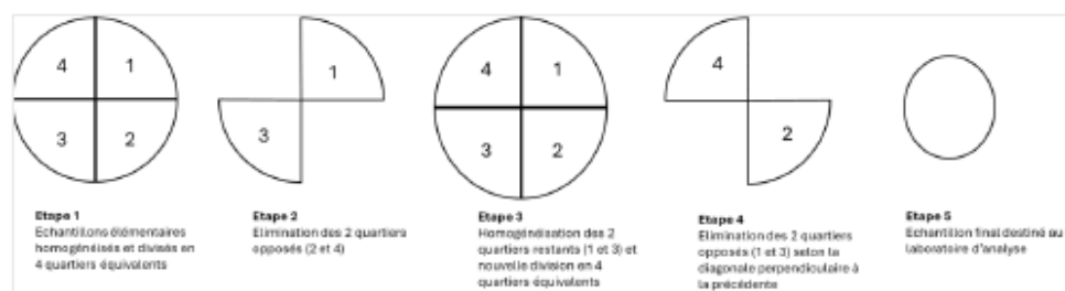
Figure 1 : Méthode de quartage
