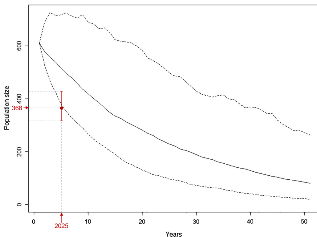
Figure 10. Prédiction de la taille médiane de la population d'Iguane des Petites Antilles de l'îlet Chancel pour les 50 prochaines années (à partir de 2021) en utilisant le taux de recrutement actuel (ligne noire avec en pointillés noirs l'intervalle de confiance à 95%) (d'après Warret Rodrigues et al, 2021) et positionnement approximatif de l'estimation 2025 de la taille de la population (en rouge).
